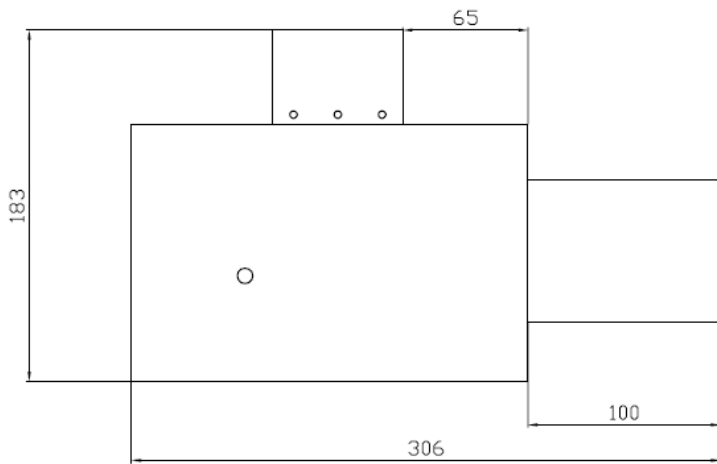
УДЛИНЕННАЯ ГОРЕЛКА
